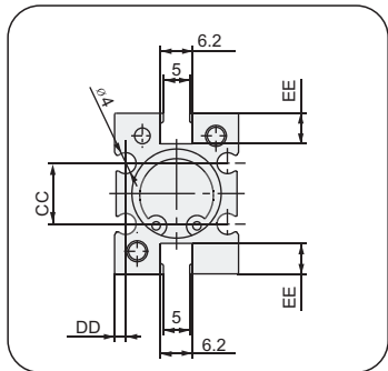
GMHZL2-□□磁性开关安装槽尺寸 GMHZL2-□□Magnetic Switch Mounting Groove Dimensions
